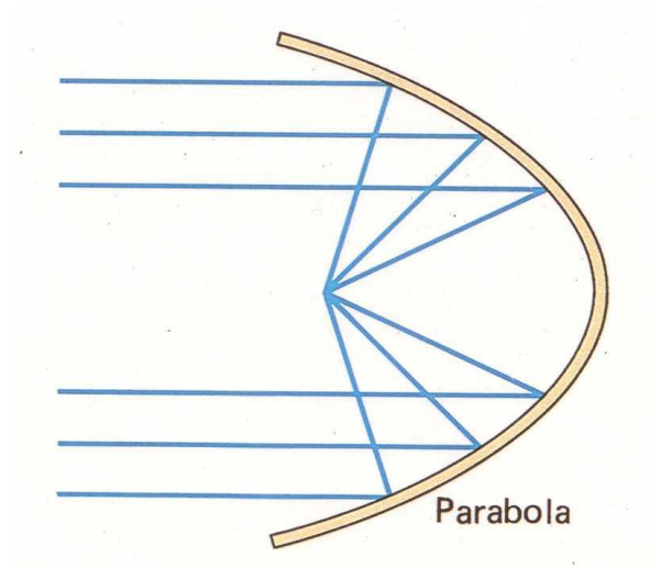
Zwierciadło paraboloidalne
